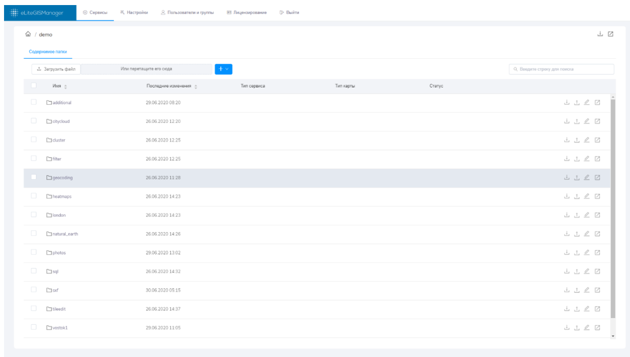
Рисунок 3 – Каталог сервисов
