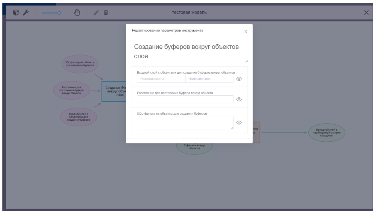
Рисунок 47 – Редактирование инструмента
