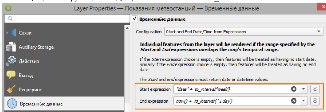
Рисунок 100 - Настройка границ временного интервала при помощи выражения
