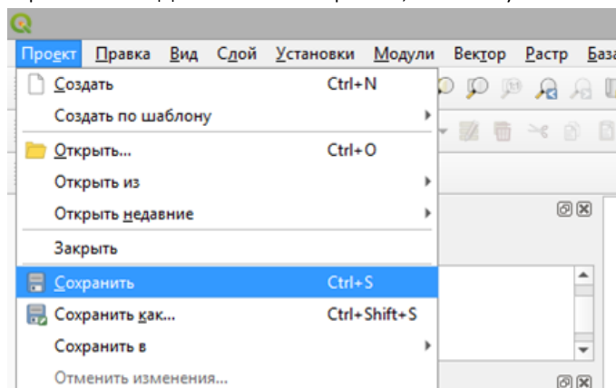
Рисунок 173 – Сохранение QGS-проекта
