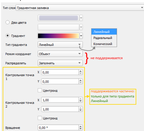
Рисунок 39 – Градиентная заливка
