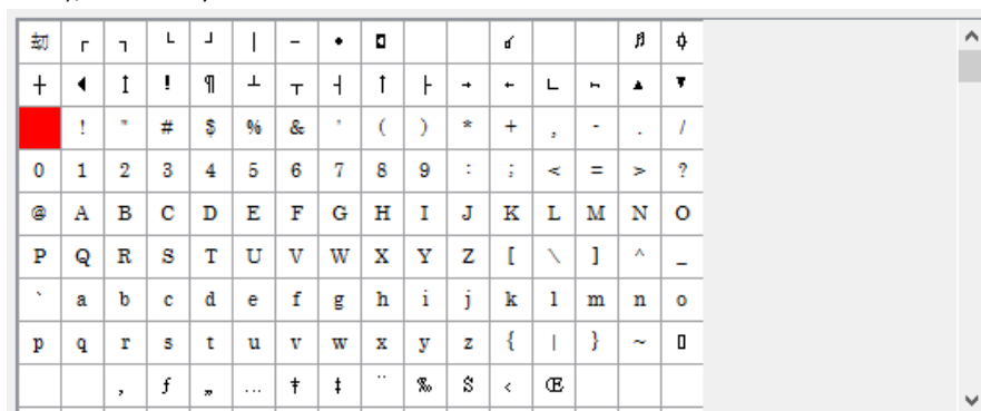
Рисунок 29 – Символьный маркер
