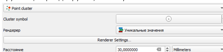
Рисунок 49 – Кластеризация
