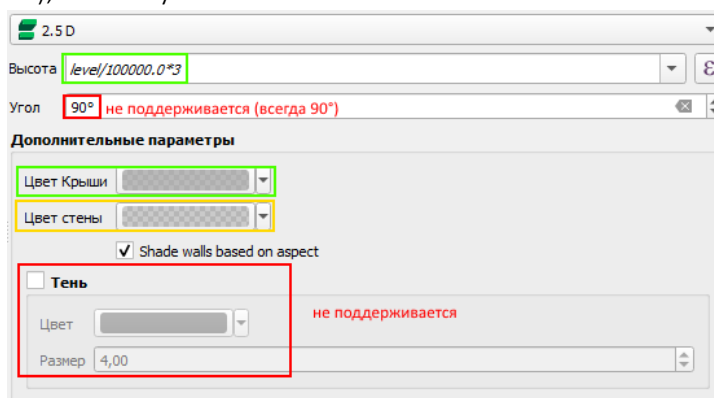
Рисунок 57 - 2.5(D) Псевдообъем
