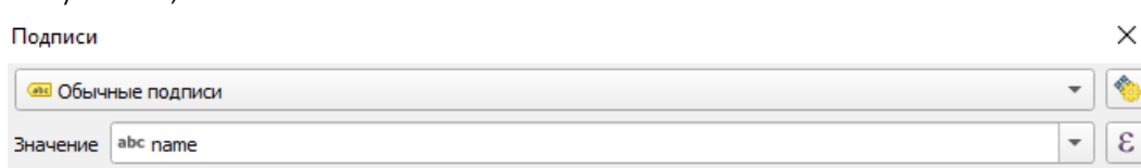
Рисунок 58 – Обычные подписи
