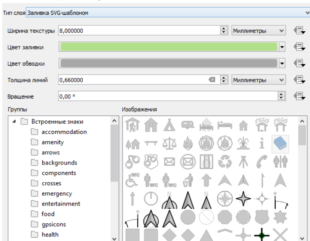
Рисунок 38 – Заливка SVG-шаблоном
