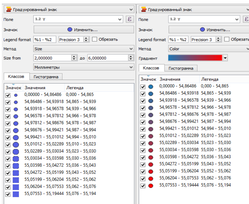
Рисунок 46 – Градуированный знак
