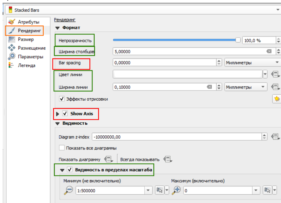
Рисунок 79 - Настройка рендеринга составных прямоугольников
