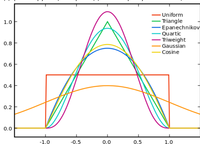
Рисунок 135 – Графики ядерных функций для использования при отрисовке термокарт
