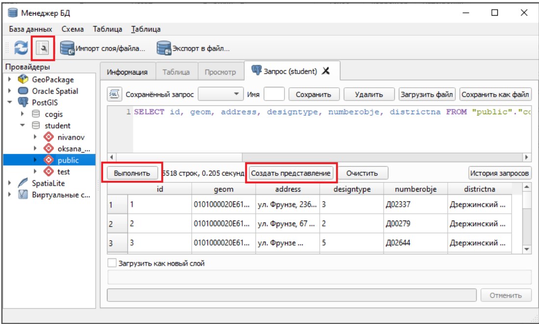
Рисунок 176 – Создание Представления (SQL-view) в Менеджере БД
