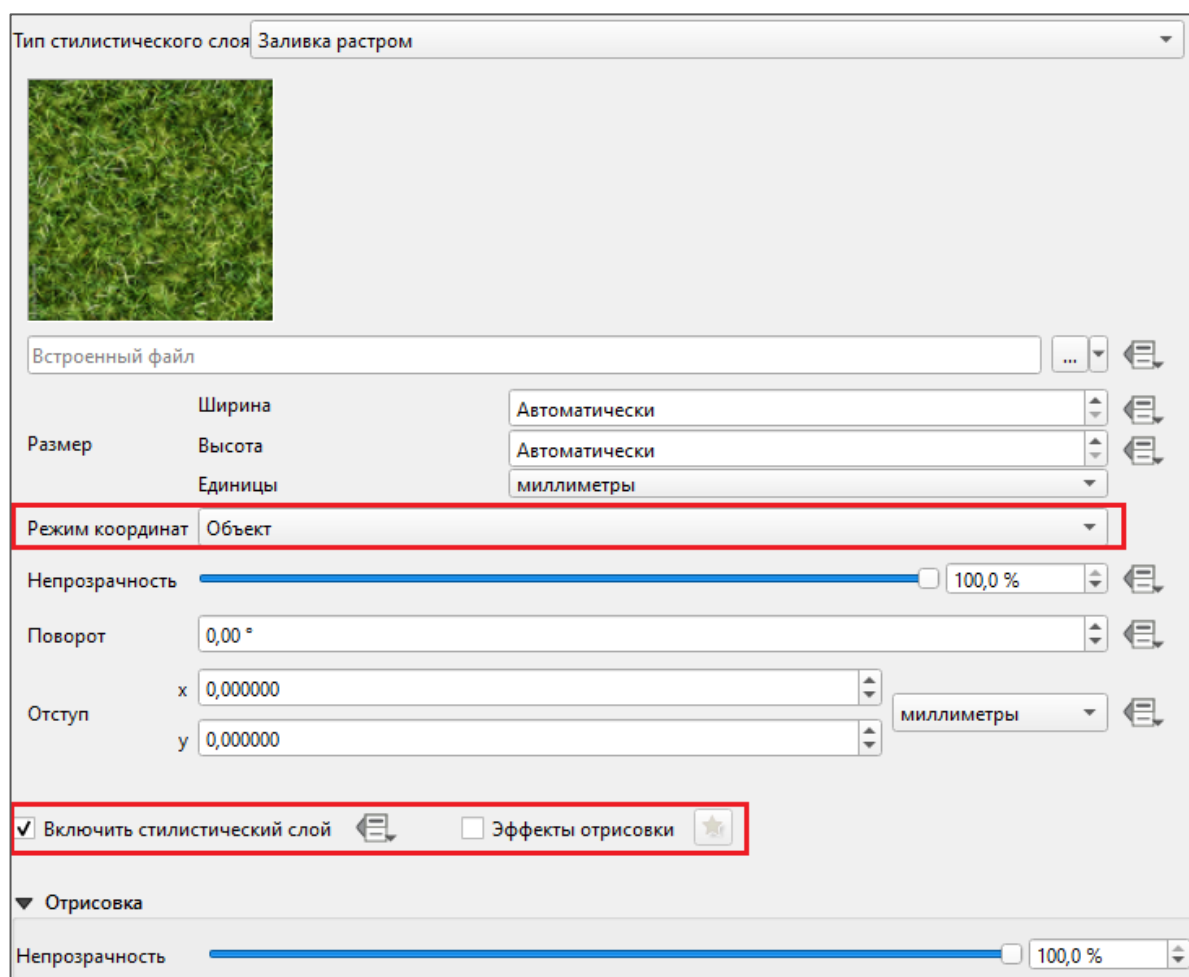
Рисунок 48 – Заливка растром (красной рамкой выделены неподдерживаемые опции: Режим координат используется всегда Объект)
