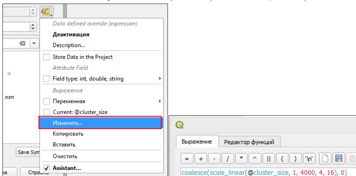
Рисунок 129 – Настройка размера кластерного символа (4)
