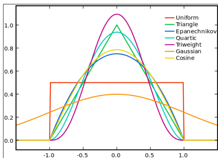
Рисунок 160 – Графики ядерных функций для использования при отрисовке тепловых карт
