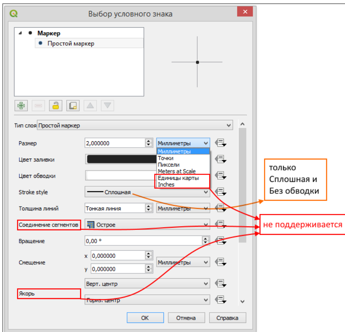
Рисунок 35 – Настройка условного знака для слоя
