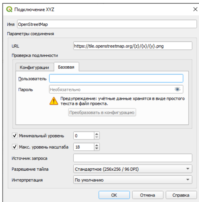
Рисунок 28 – Создание подключения XYZ для добавления тайлового слоя OpenStreetMap к картографическому проекту
