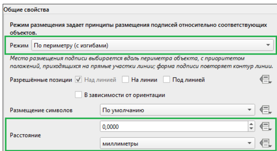
Рисунок 88 – Поддерживаемая опция Расстояние для режима По периметру (с изгибами)
