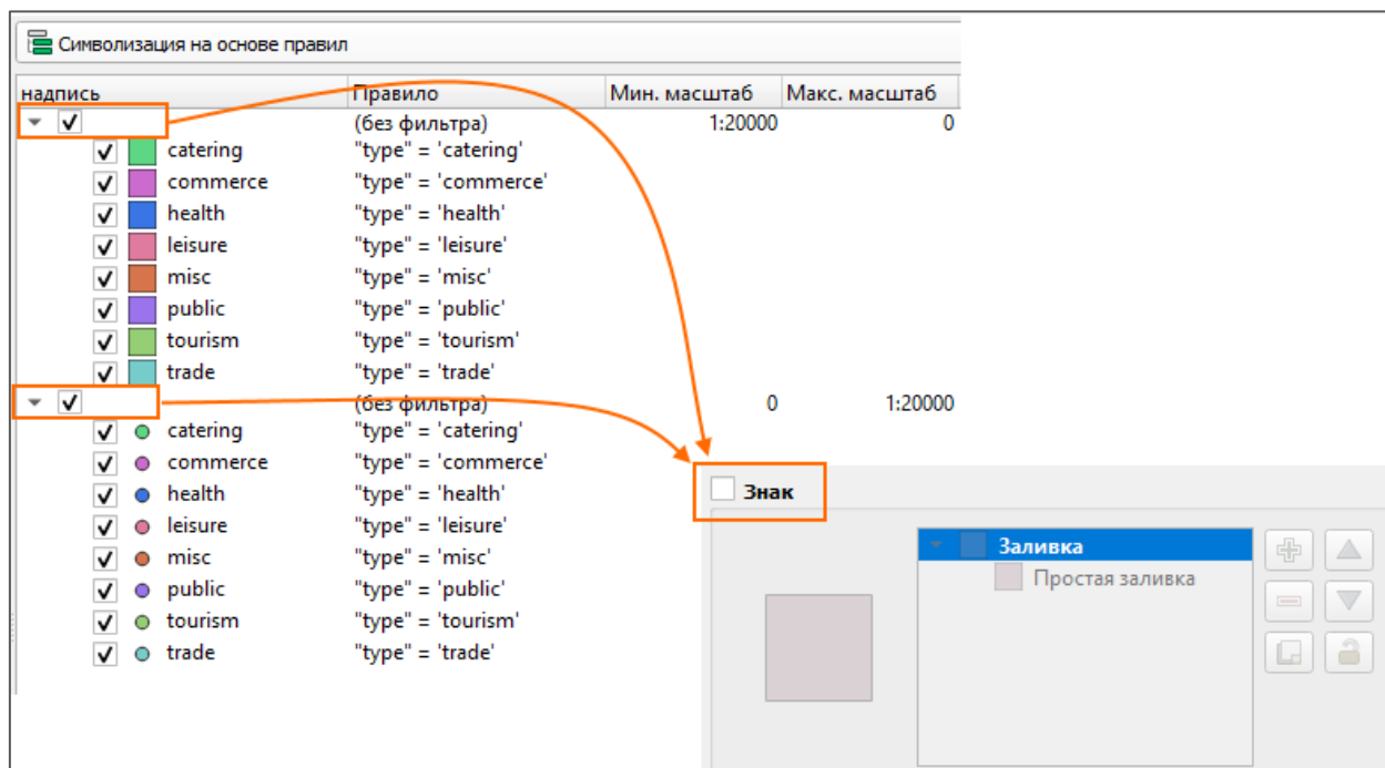
Рисунок 60 – Настройка правил отображения символов на разных масштабах
