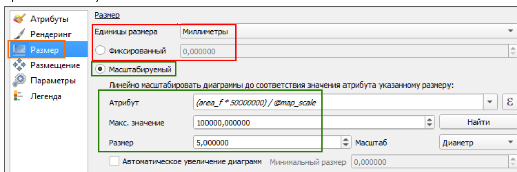
Рисунок 98 - Настройка размера составных прямоугольников
