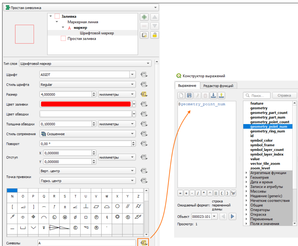
Рисунок 188 – Настройка подписи в шрифтовом маркере
