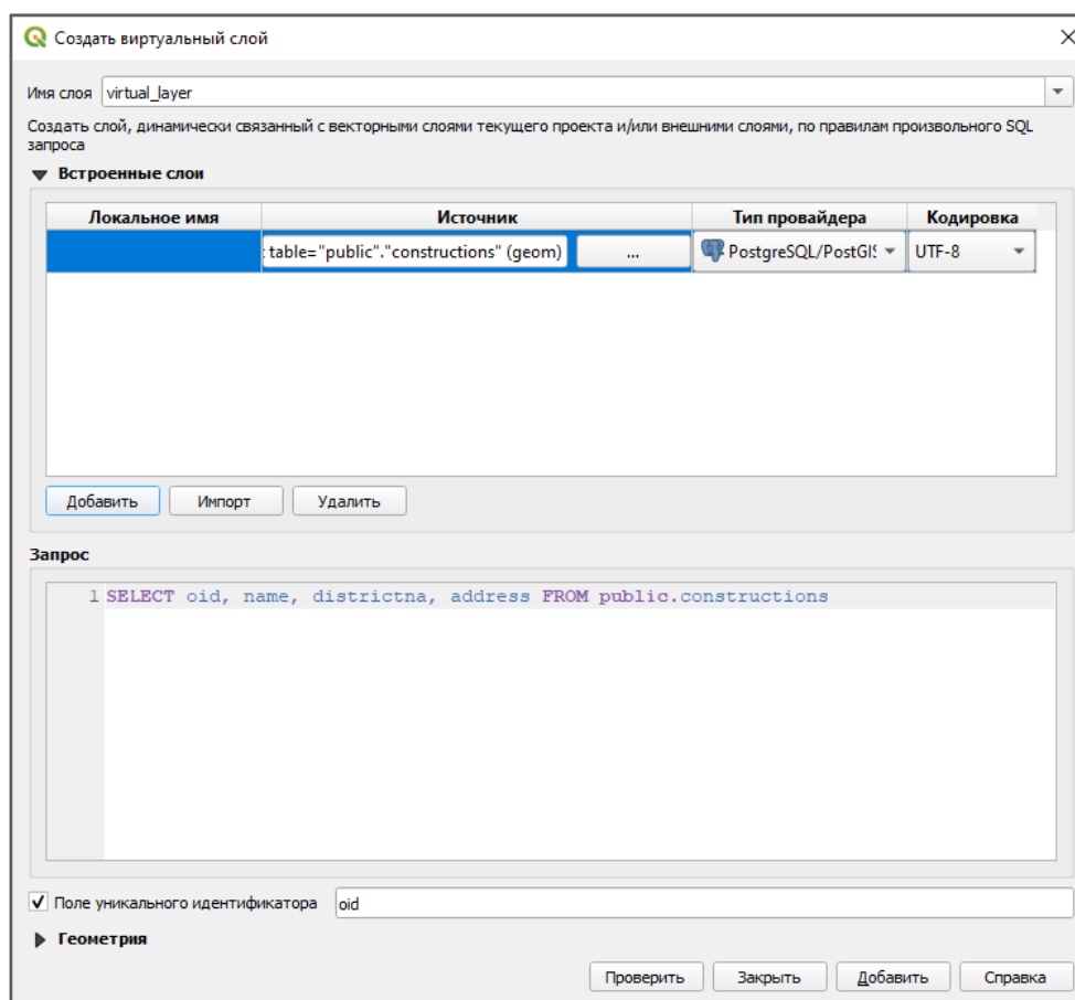
Рисунок 155 – Настройка виртуального слоя
