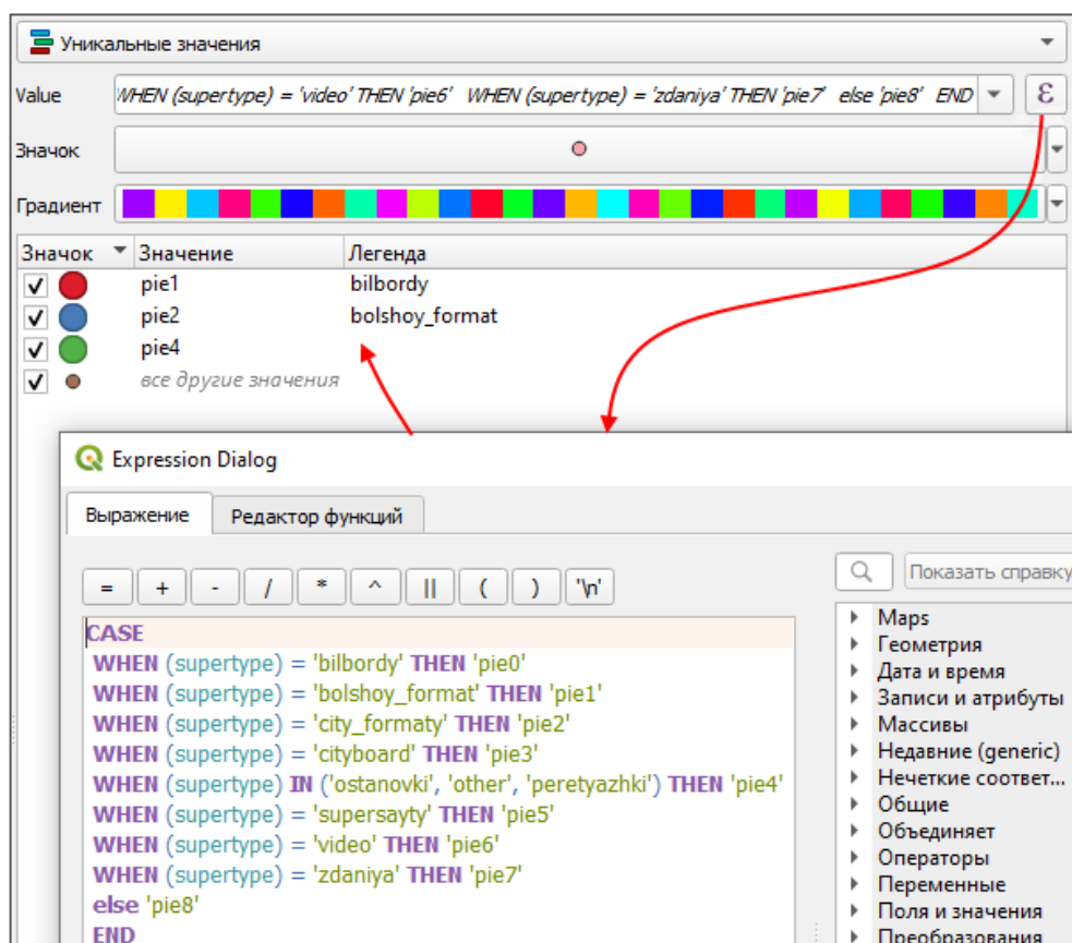
Рисунок 143 – Настройка цветов для сегментов круговой диаграммы с помощью SQL-выражений
