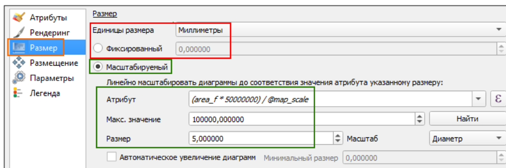
Рисунок 94 - Настройка размера круговой диаграммы
