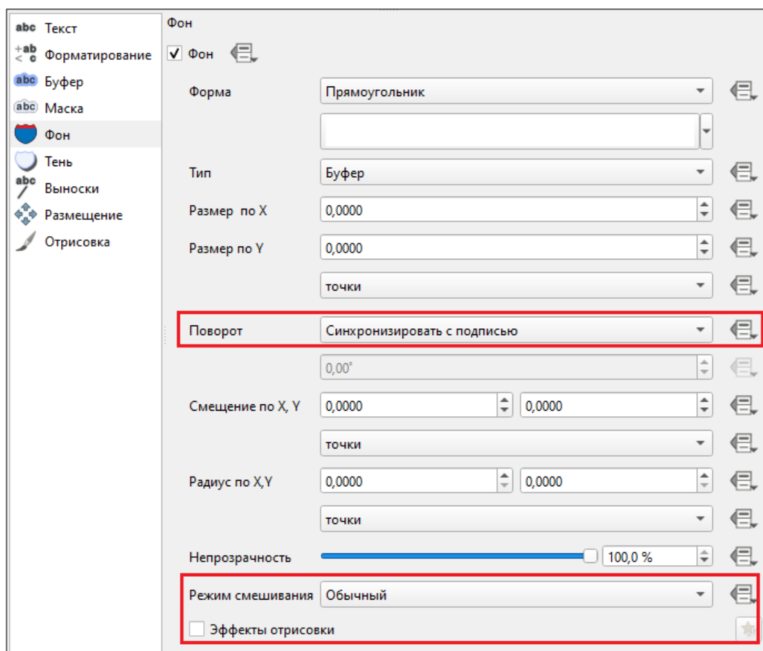
Рисунок 78 – Настройки фона для подписей (красной рамкой выделены неподдерживаемые настройки)
