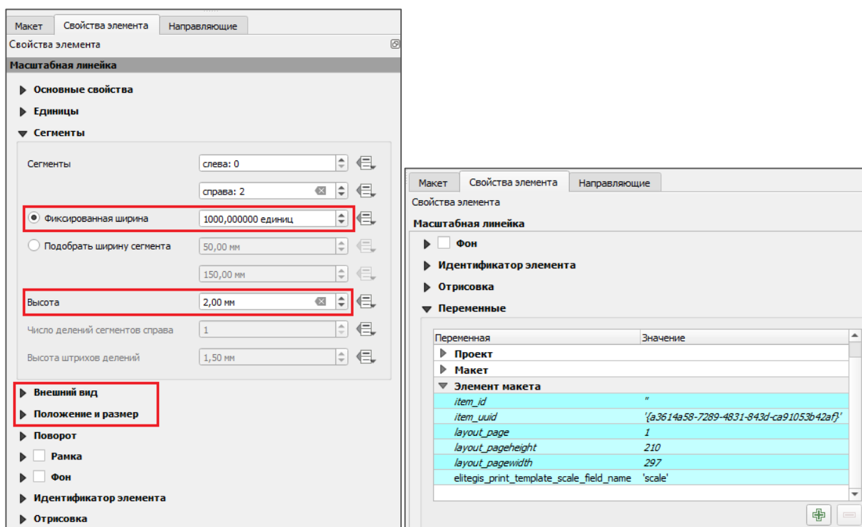
Рисунок 230 – Поддерживаемые настройки элемента Масштабная линейка
