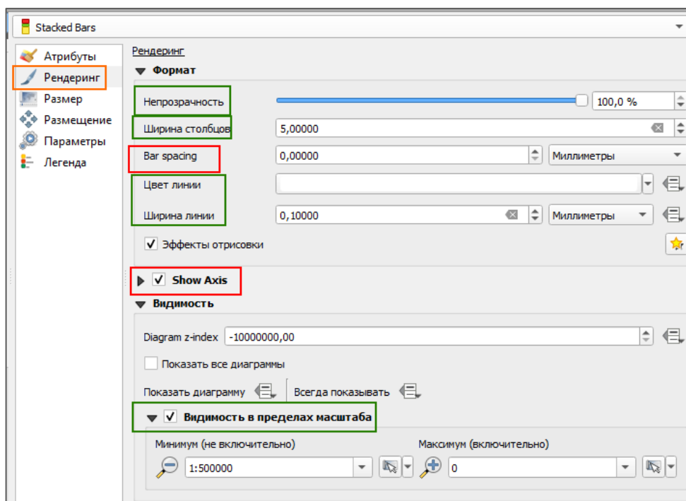
Рисунок 97 - Настройка рендеринга составных прямоугольников
