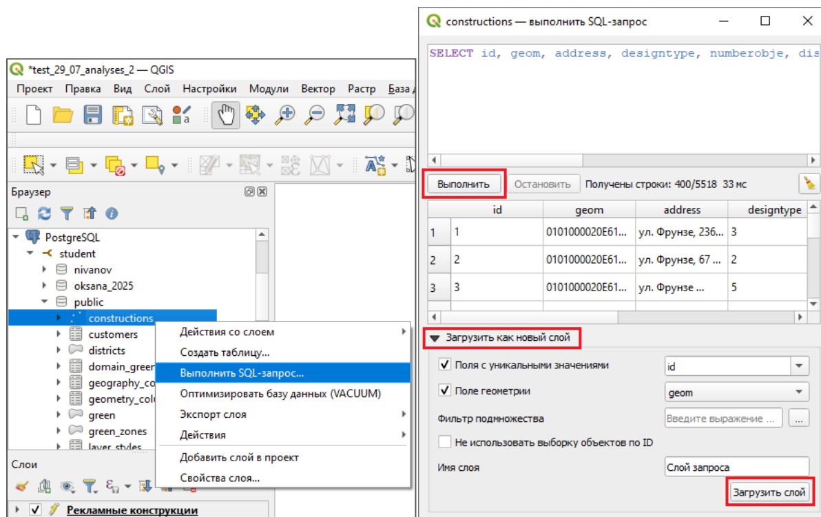
Рисунок 157 - Создание слоя запроса через команду контекстного меню таблицы в базе данных
