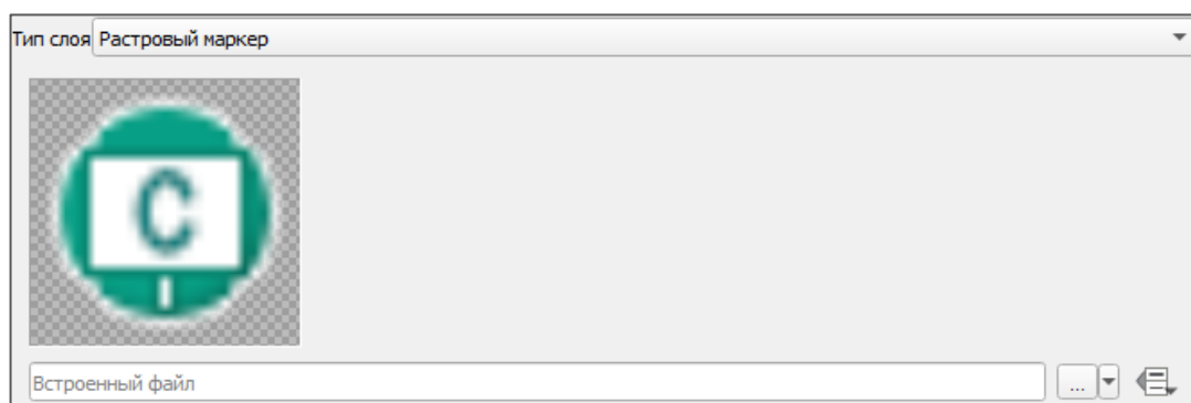
Рисунок 40 – Растровый маркер
