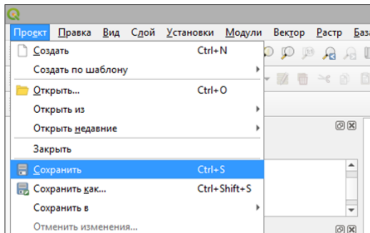
Рисунок 209 – Сохранение QGS-проекта
