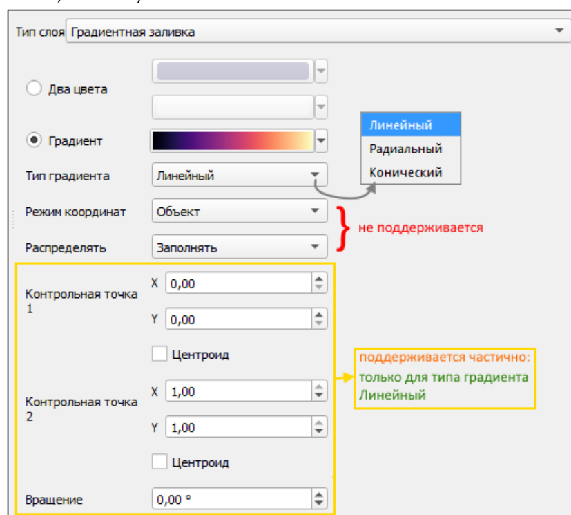
Рисунок 50 – Градиентная заливка
