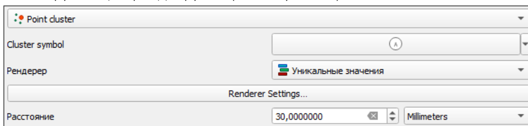
Рисунок 61 – Кластеризация
