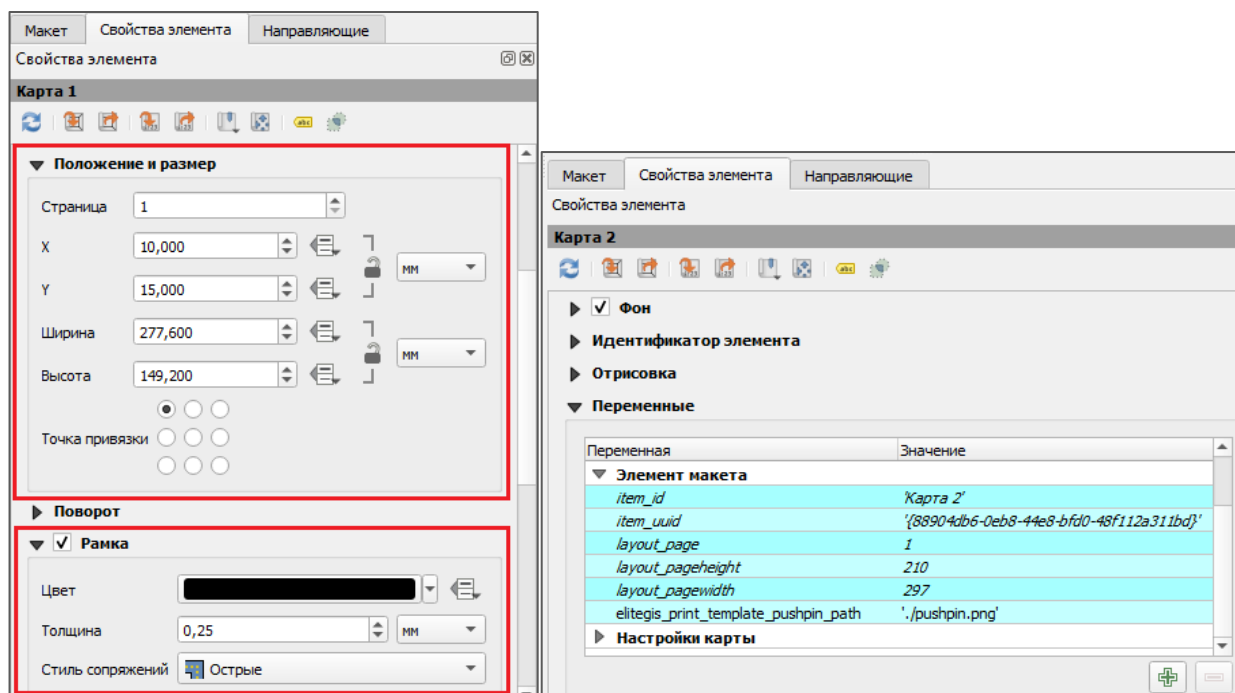
Рисунок 226 – Поддерживаемые настройки элемента Карта (Словарь)
