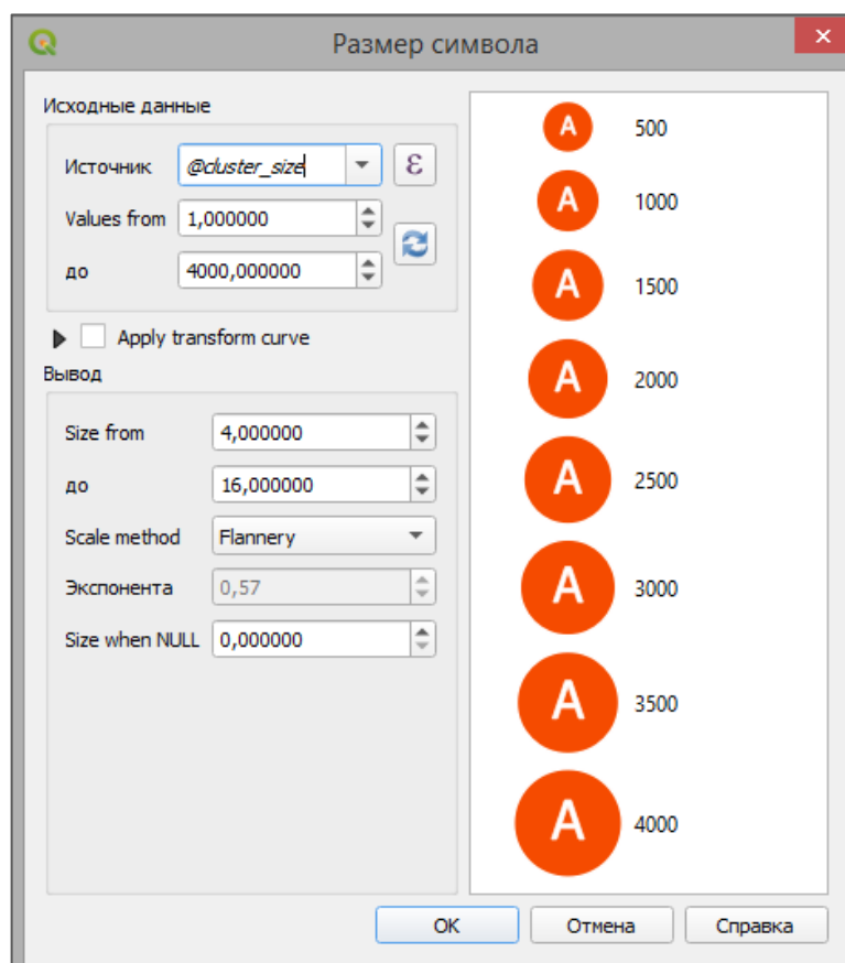
Рисунок 128 – Настройка размера кластерного символа (3)
