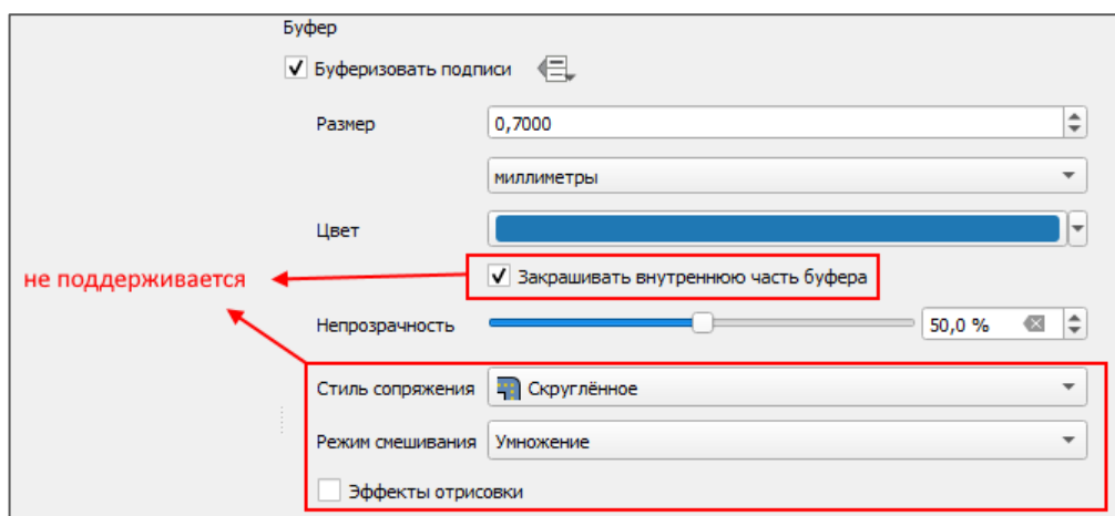
Рисунок 77 – Настройки буфера для подписей
