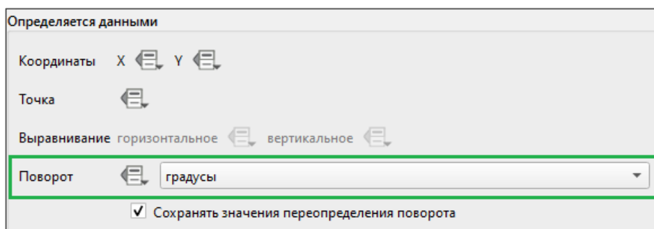
Рисунок 89 – Поддерживаемая настройка поворота подписи
