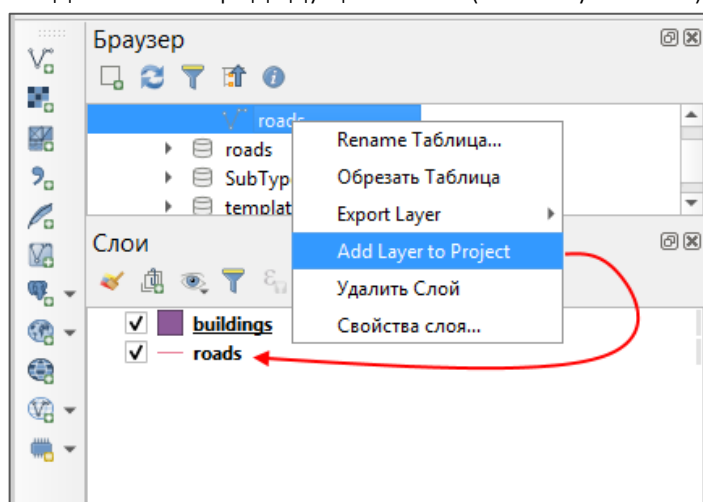
Рисунок 202 – Добавление слоев для геокодера в картографический проект QGIS
