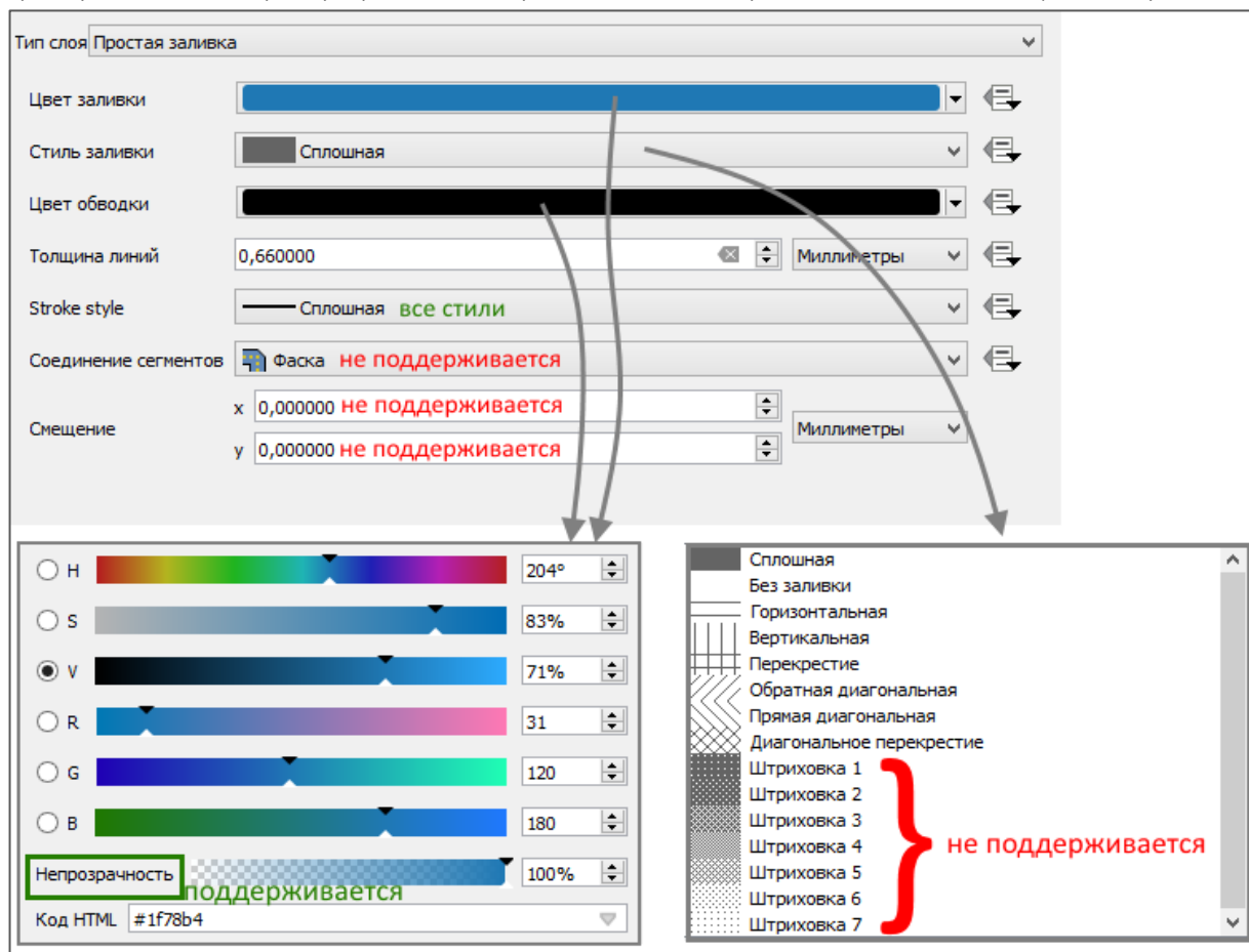
Рисунок 46 – Простая заливка
