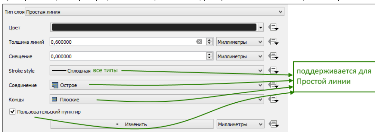
Рисунок 43 – Простая линия
