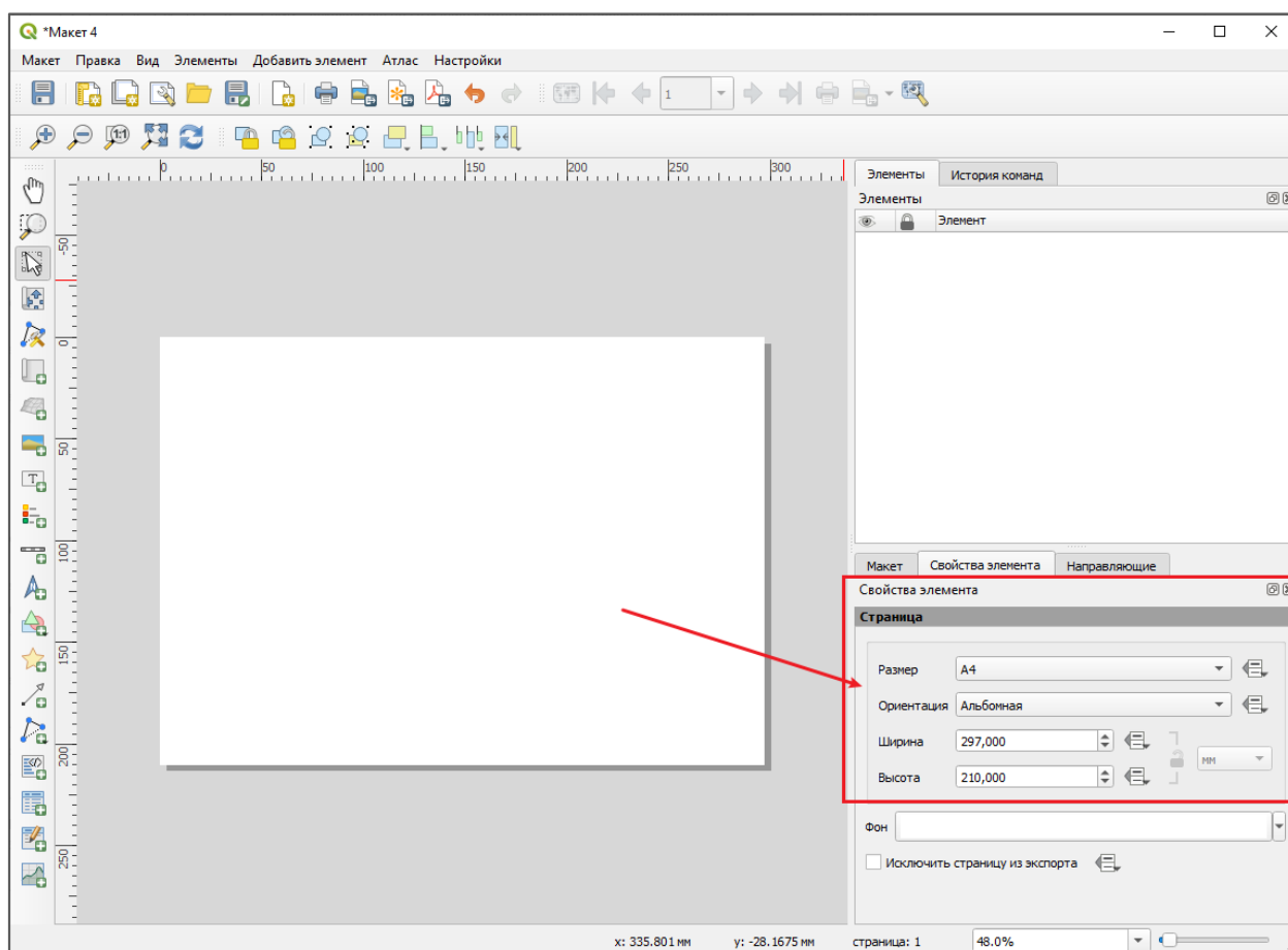
Рисунок 224 – Свойства листа
