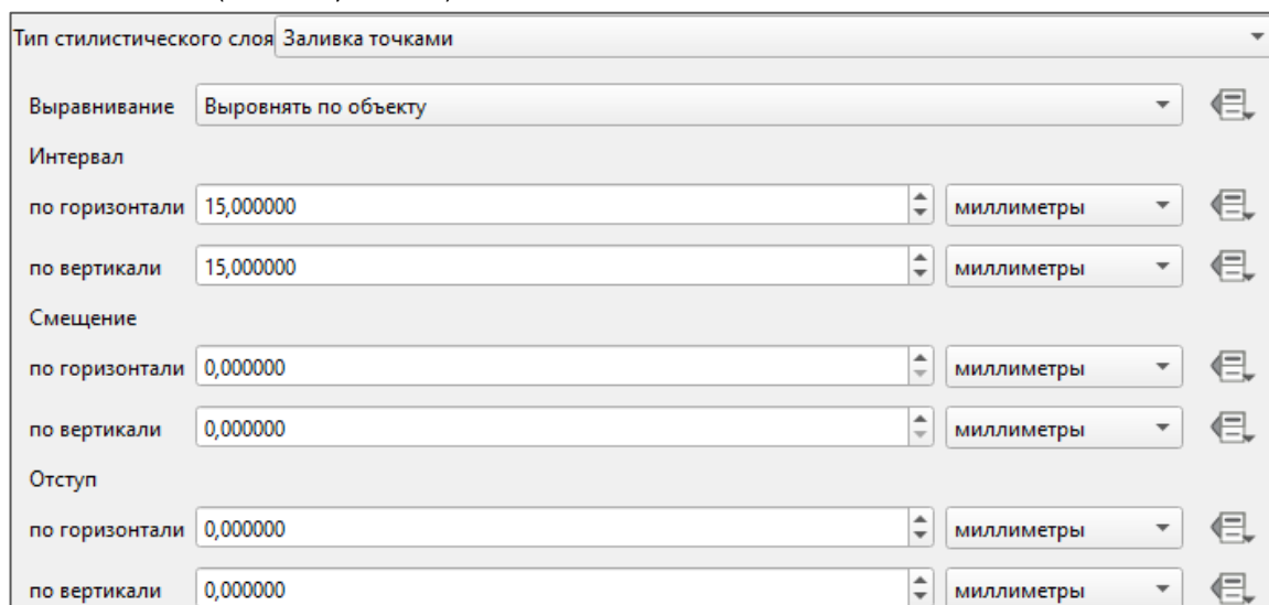
Рисунок 47 – Заливка точками
