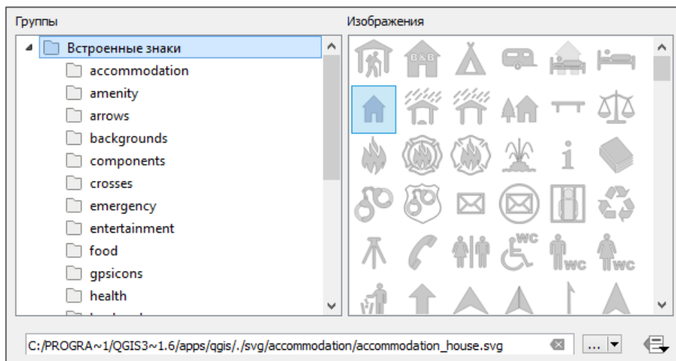
Рисунок 41 – SVG-маркер
