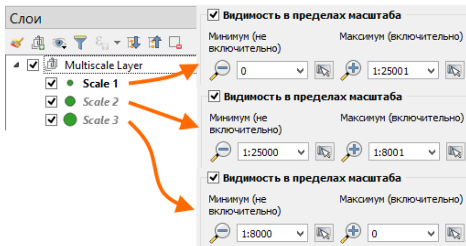
Рисунок 31 – Мультимасштабный слой
