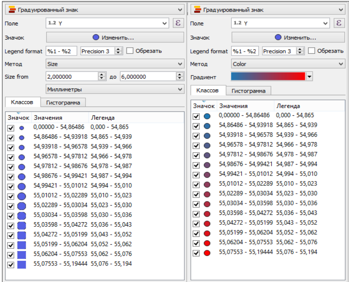
Рисунок 58 – Градуированный знак
