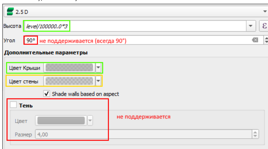
Рисунок 66 - 2.5(D) Псевдообъем
