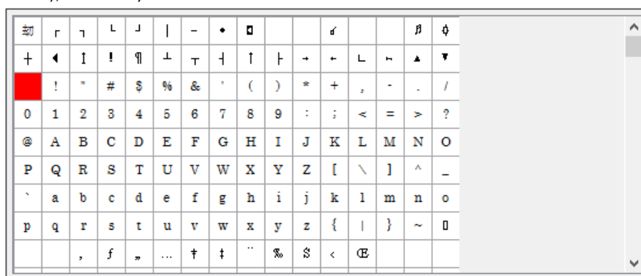
Рисунок 39 – Шрифтовой маркер
