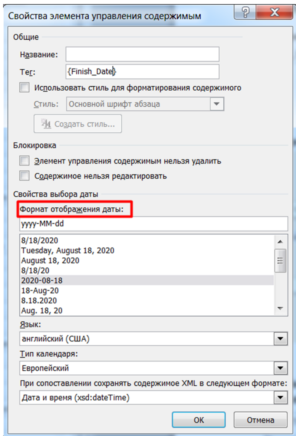
Рисунок 202 – Формат отображения даты
