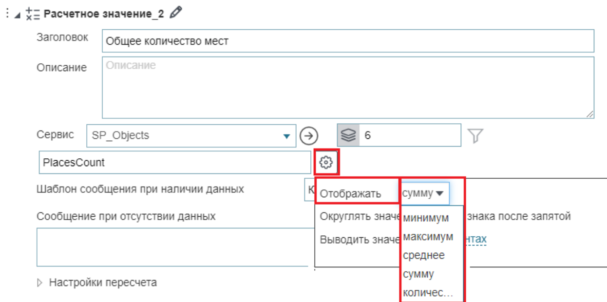
Рисунок 161 – Выбор статистического показателя
