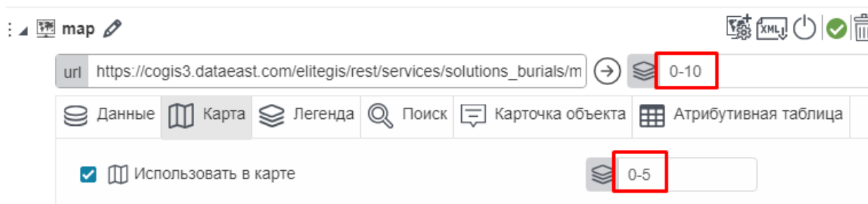
Рисунок 217 – Пример настройки слоев для скачивания на устройство в мобильном приложении
