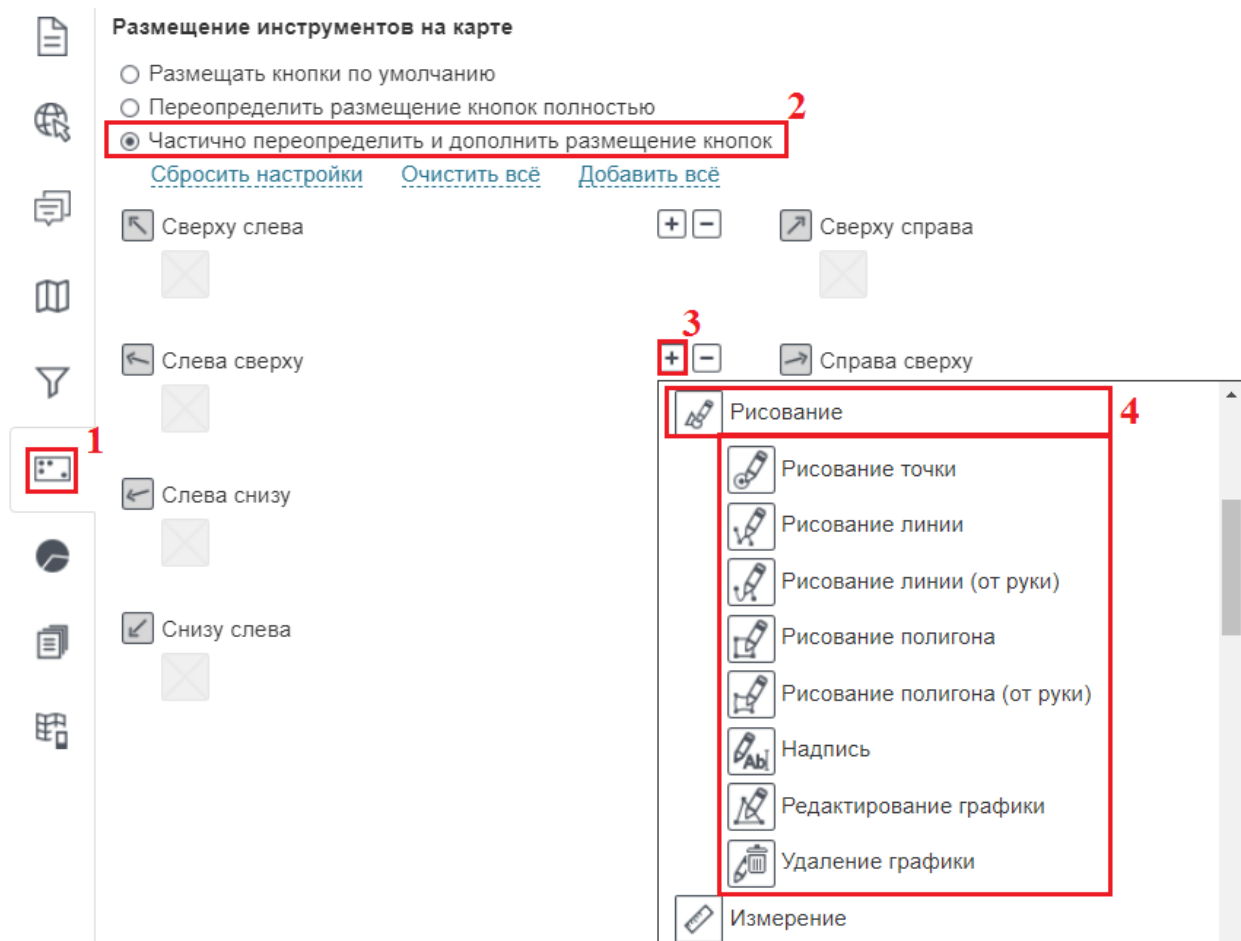
Рисунок 97 – Размещение инструментов на карте
