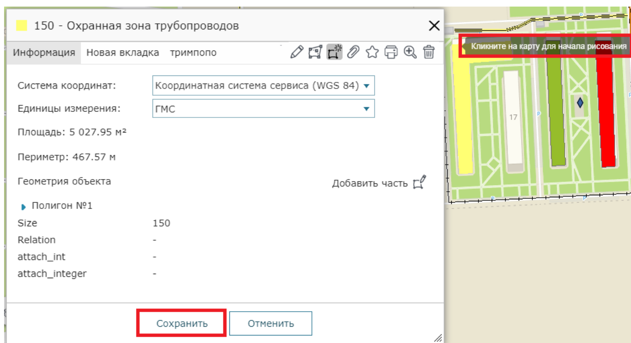
Рисунок 66 – Сохранение изменений после редактирования геометрии объекта полигонального слоя
