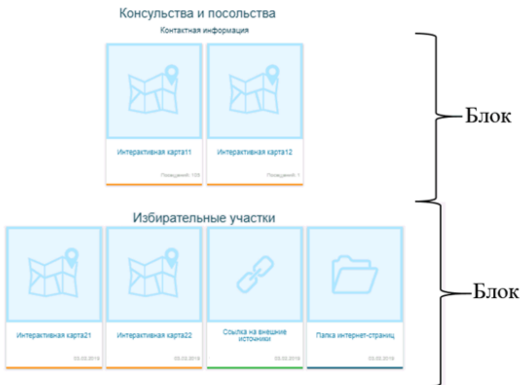
Рисунок 13 – Папка в виде блока
