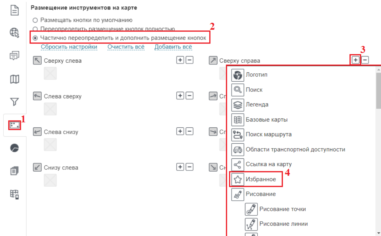
Рисунок 77 – Размещение инструментов на карте
