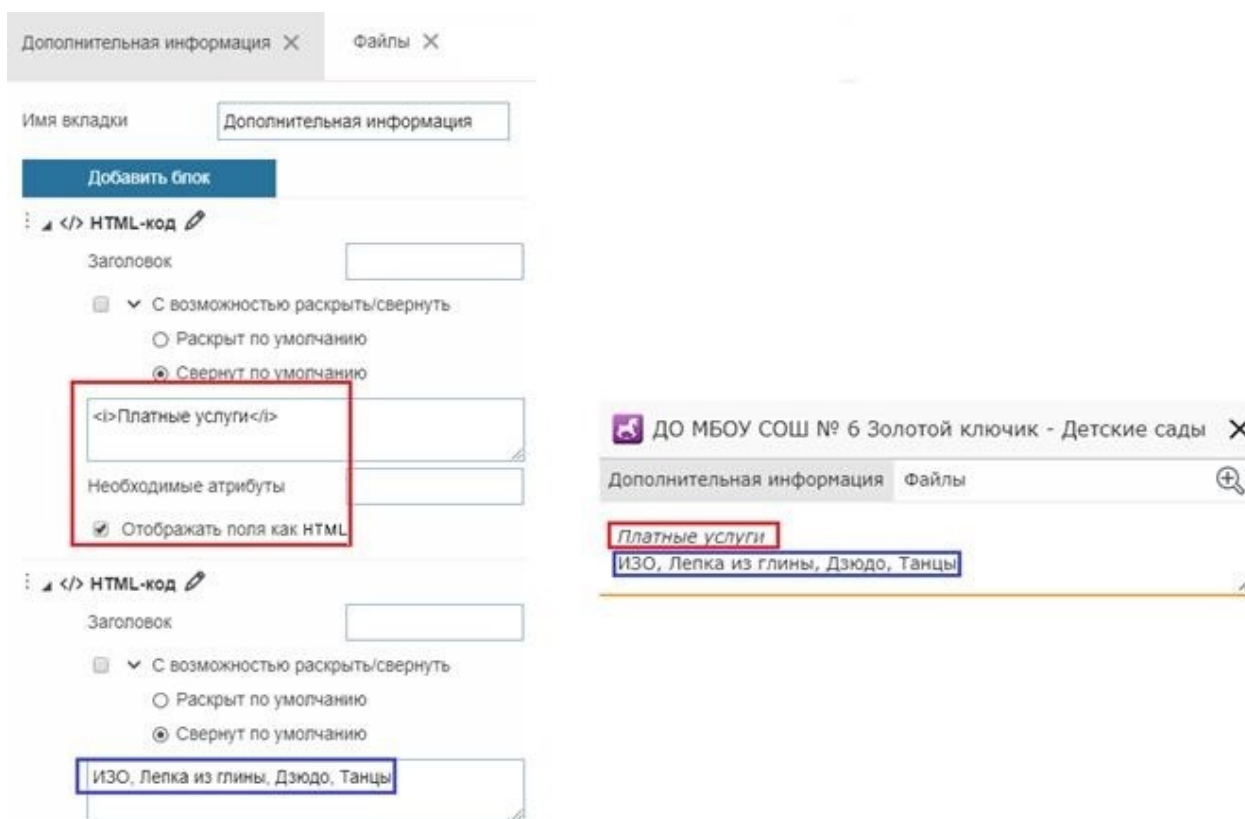
Рисунок 73 – Отображение блока «HTML-код»
