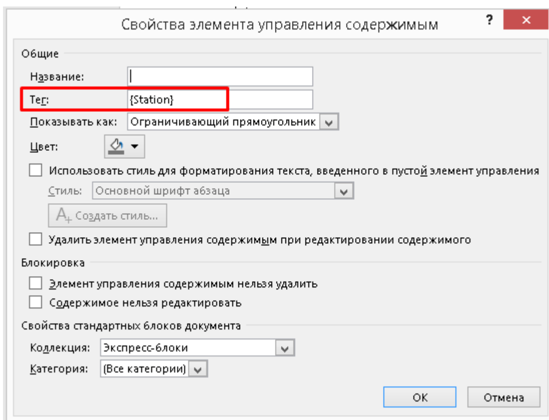
Рисунок 199 – Вставка значения параметра в отчет
