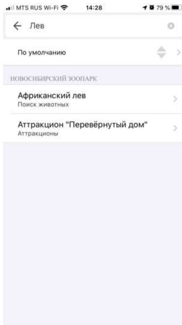
Рисунок 9 – Результаты поиска
